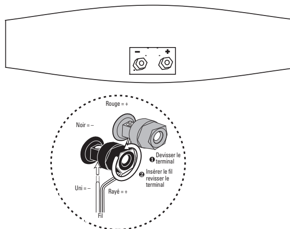
Figure 5. Les borniers des enceintes satellites et de l'enceinte centrale peuvent être connectés de plusieurs façons, par exemple avec cosse ou fils nus (comme sur l'illustration).
